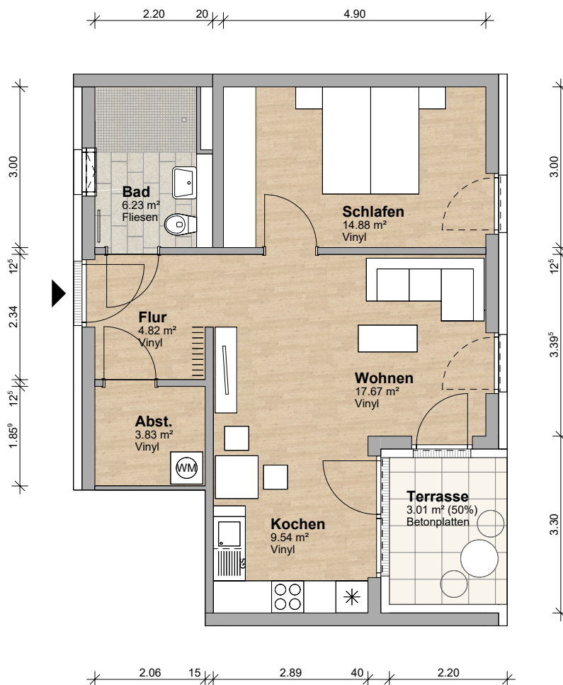
Grundriss M 1:100
